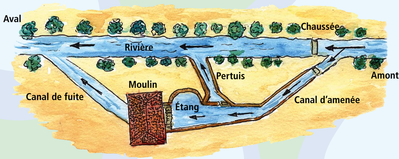
Bief (vue de dessus)
